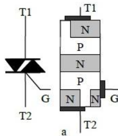
图 1 三端双向交流开关原理图
