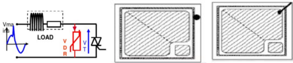
图 2 测试原理图
