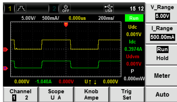
图 13 IT6400 面板波形图
