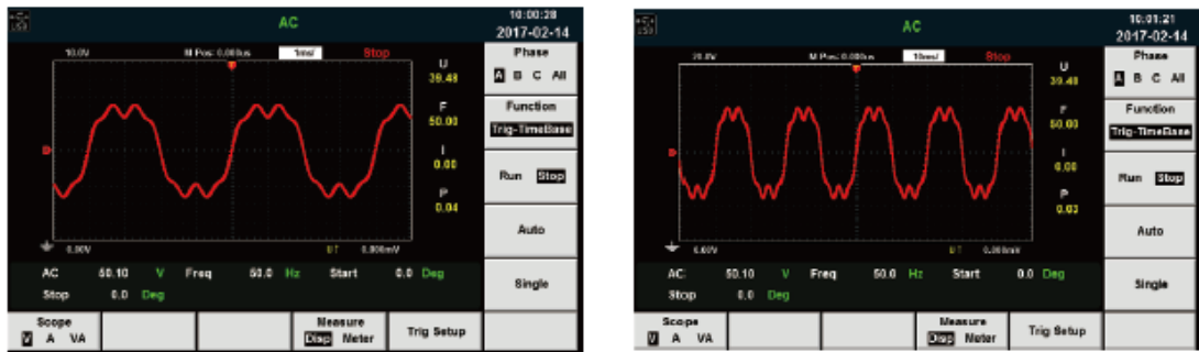
图 8 IT7600 面板波形图
