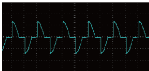
前沿相位调光
