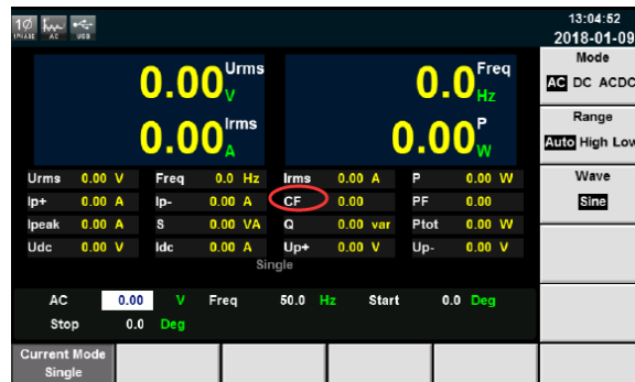
图 9 IT7600 面板图
