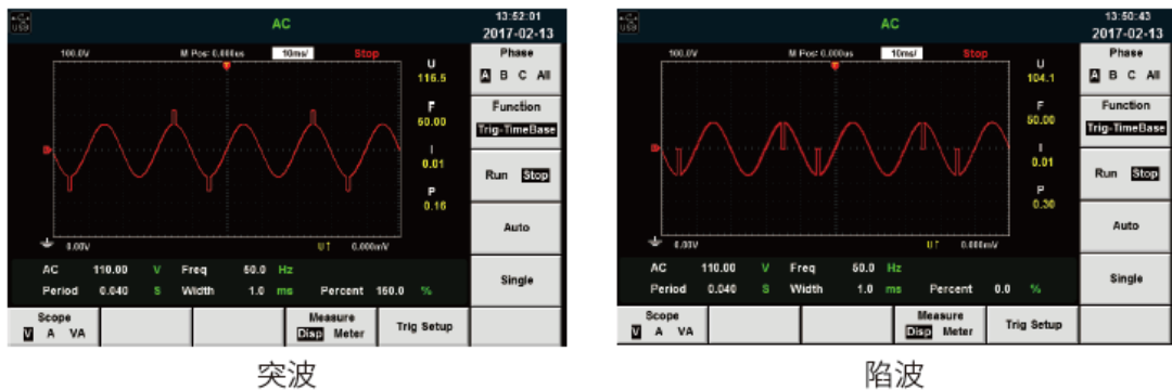
图 5 IT7600 面板波形图
