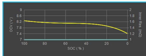
Ni/MH
